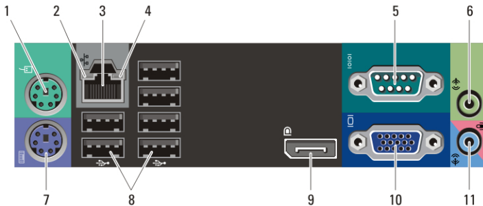
Slika 5. Prikaz zadnje ploče za Mini-Tower i Desktop kućišta
