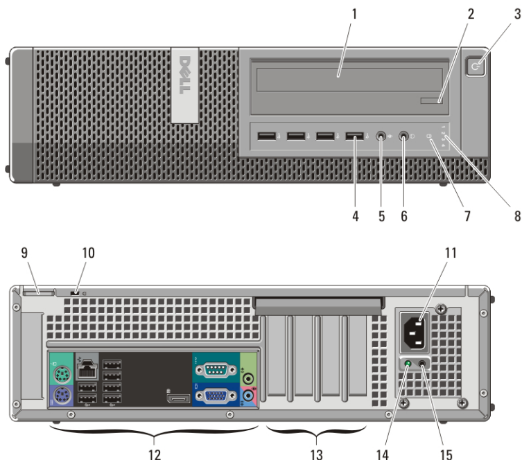
Slika 2. Prikaz sa prednje i zadnje strane za Desktop kućište
