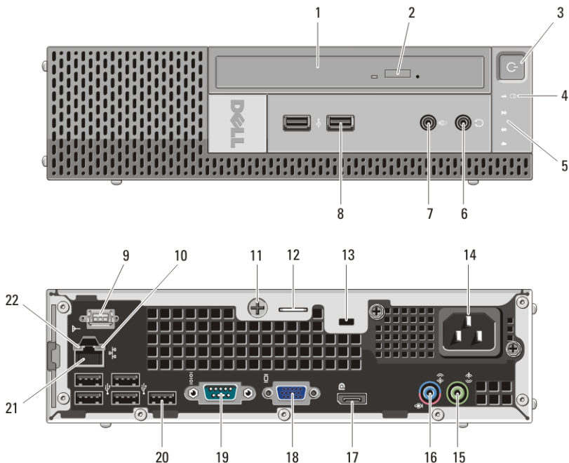
Slika 4. Prikaz sa prednje i zadnje strane za Ultra Small Form Factor kućište
